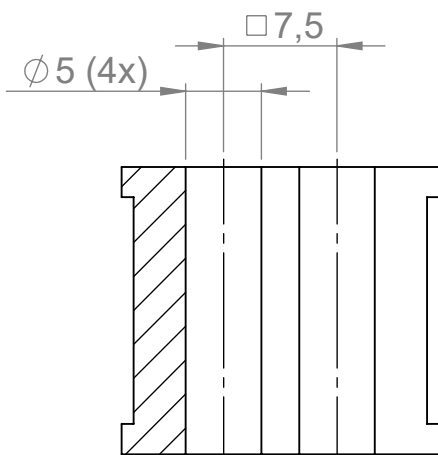
SCHNITT A-A
