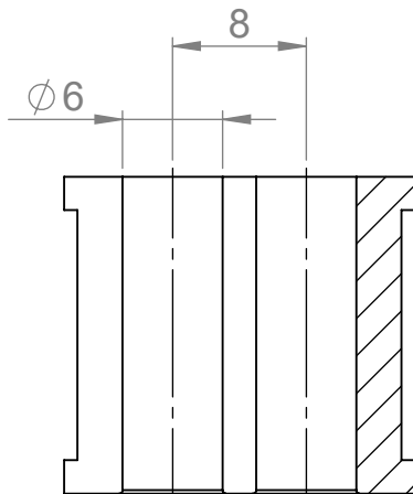
SCHNITT A-A
